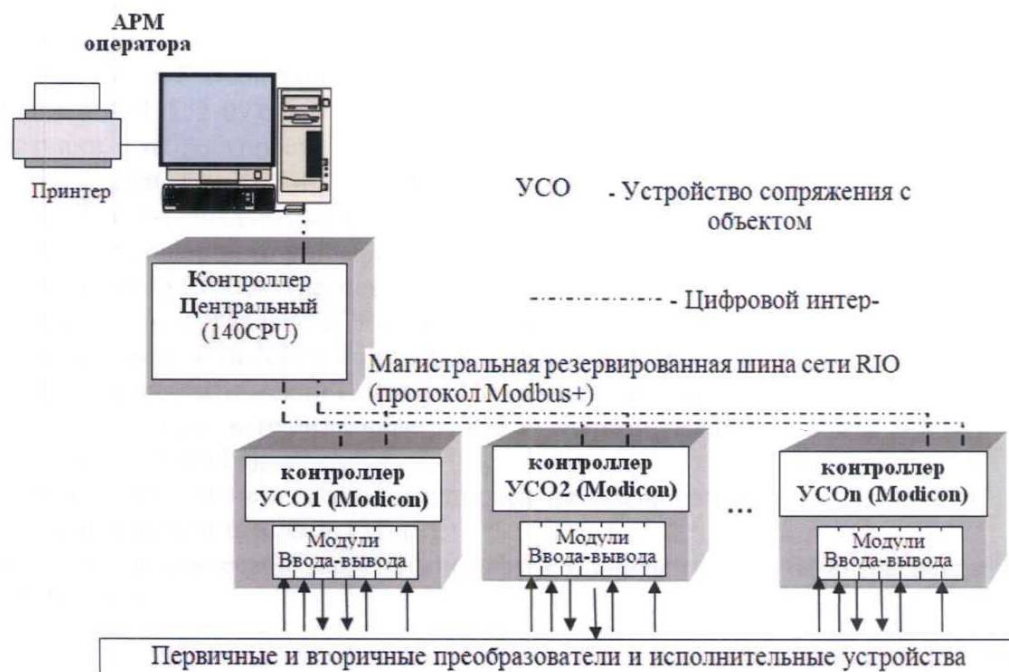
Рисунок 2 - Структурная схема ИС-ЭМИКОН на базе контроллеров Modicon
